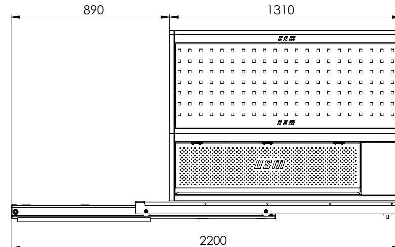
Vista lateral extendido
