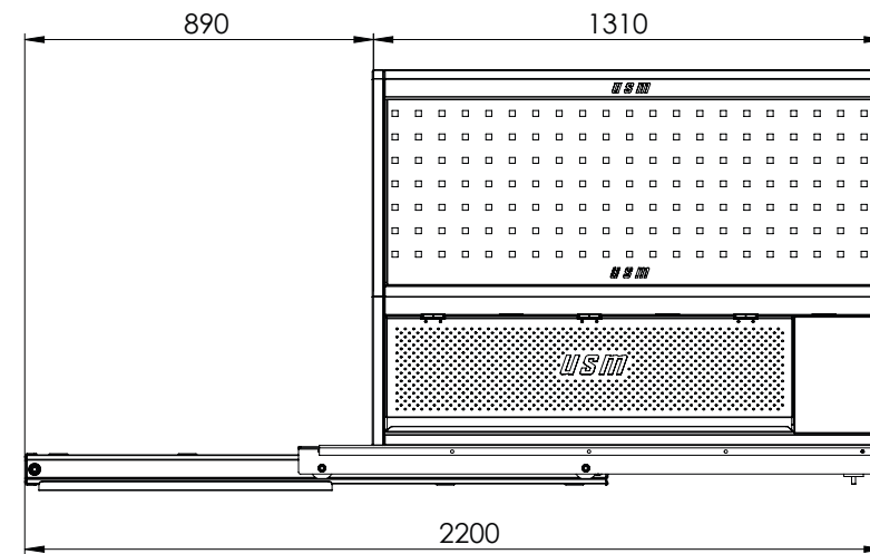
Vista lateral extendido
