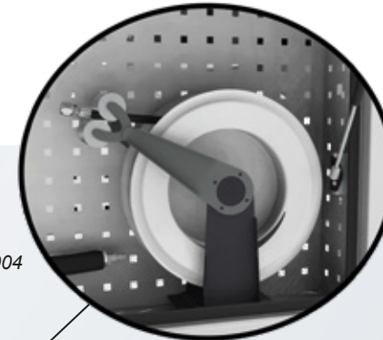
Enrollador de aceite retractil con acople rápido.
