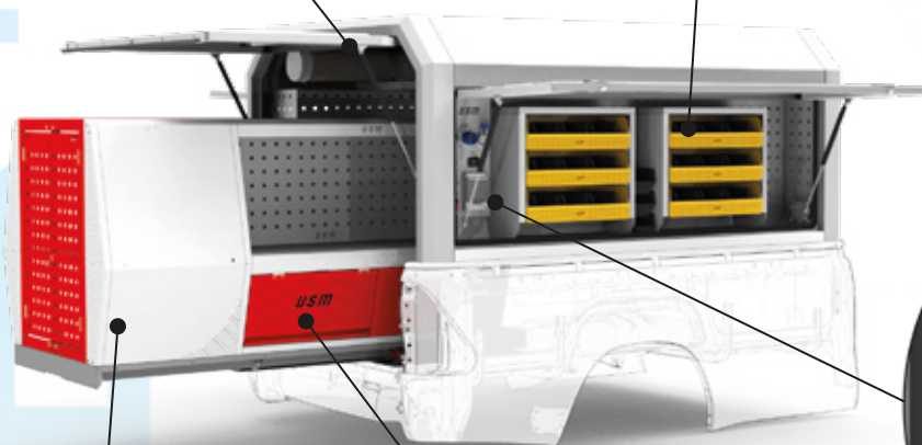
Módulo de Servicio extraíble.
