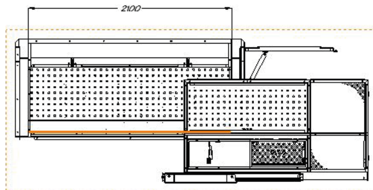
SECCIÓN H-H
